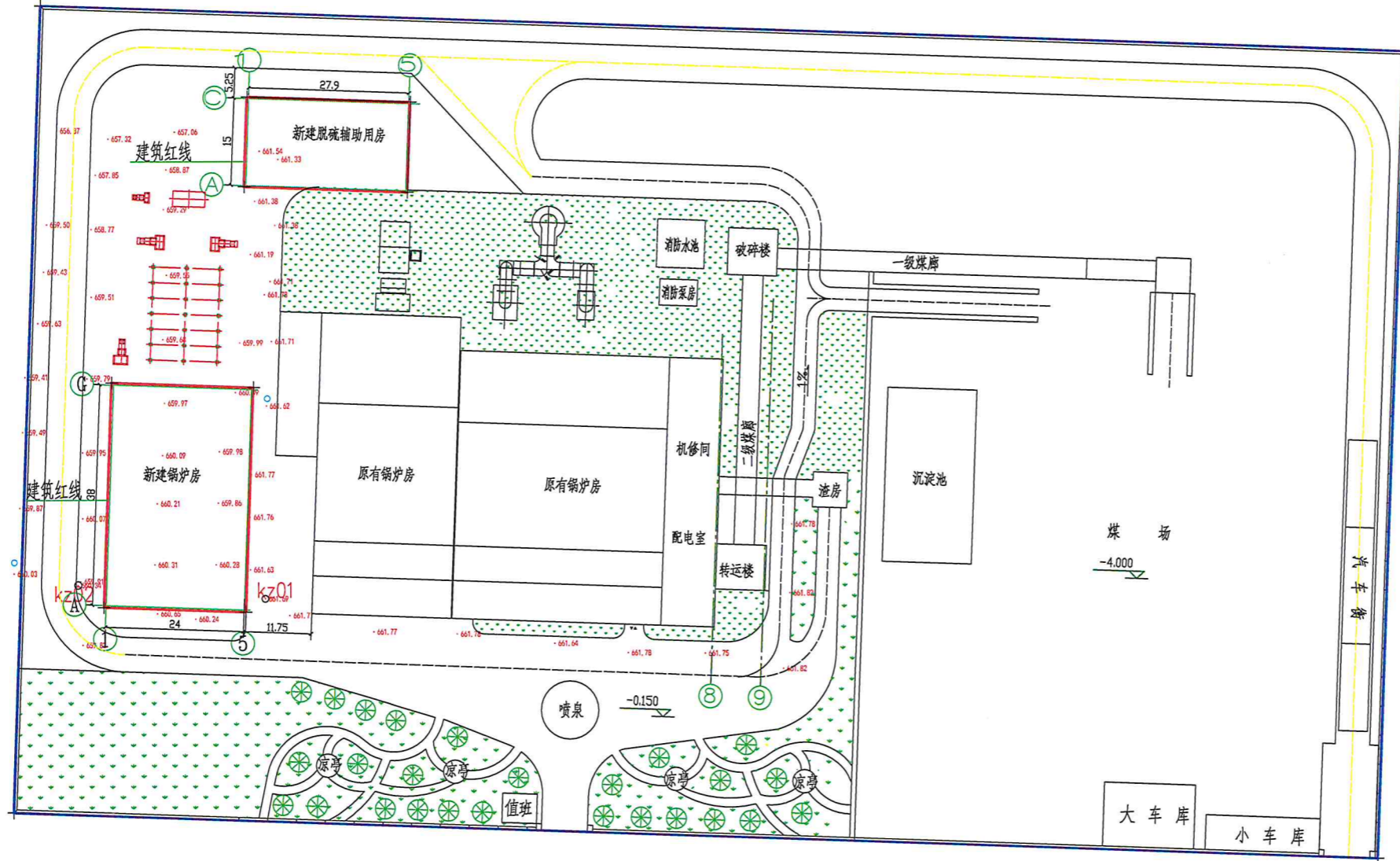
总平面布置图不带坐标 1:500
